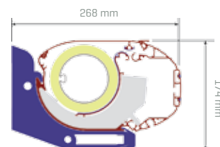
Montage contre les chevrons de toiture consols de chevron de toiture*
