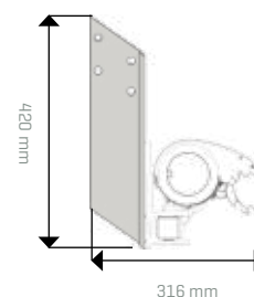
Montage contre les chevrons de toiture consoles de chevron de toiture*
