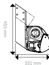
Montage au plafond étriers de plafond*
