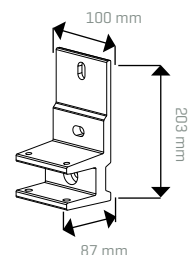
Montage contre les chevrons de toiture consoles de chevron de toiture*
