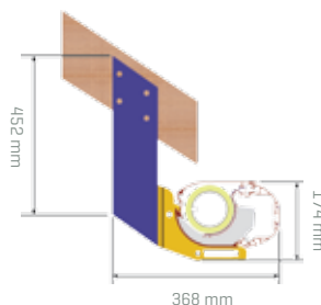
Montage au plafond étriers de plafond*
