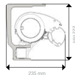
Montage contre les chevrons de toiture consoles de chevron de toiture*
